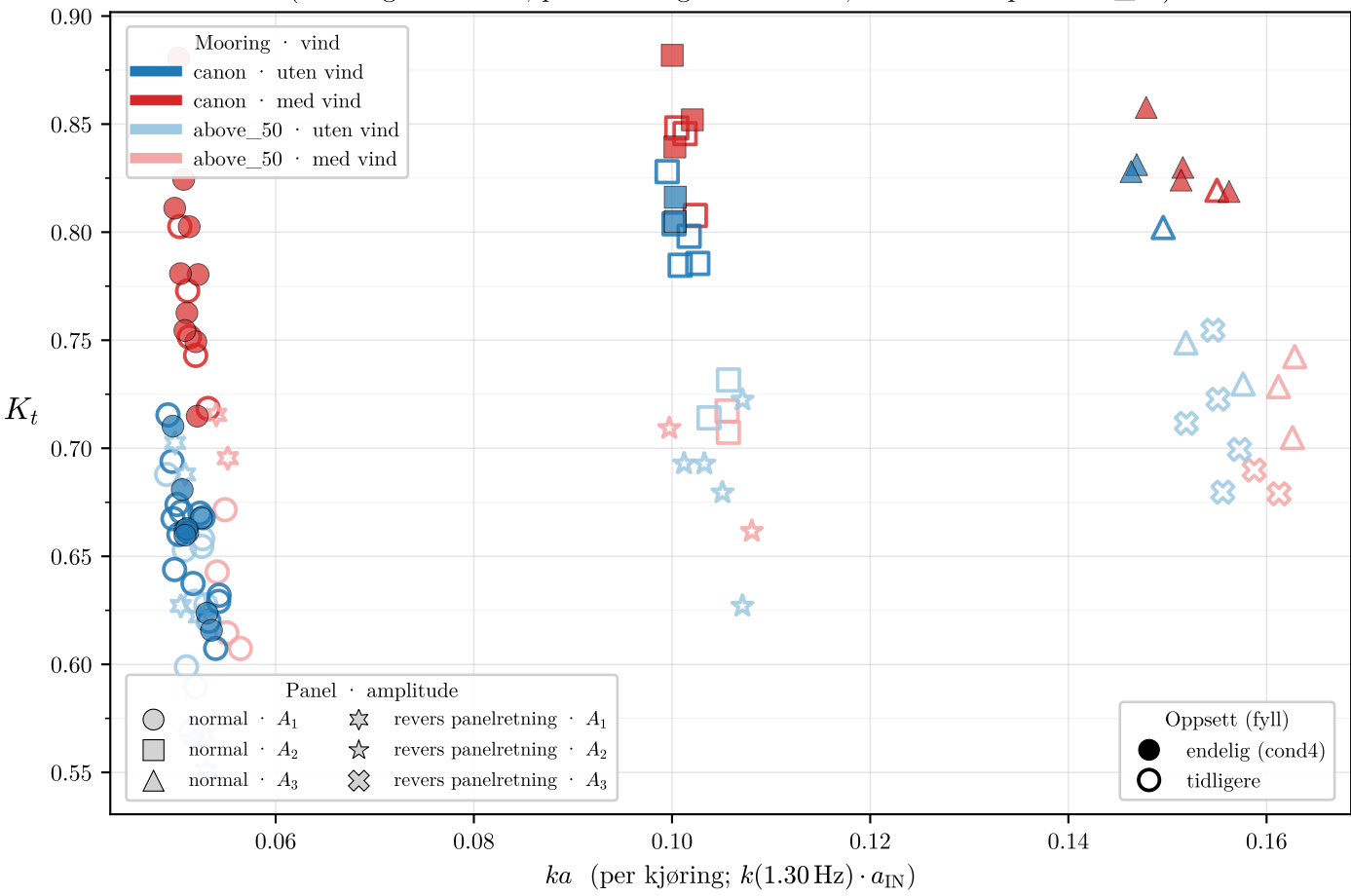
Mooring og panelretning ved 1.3 Hz — K_t vs ka (mooring dominerer; panelretning er sekundær, kun målbar på above_50)
